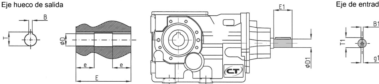
Eje hueco de salida
