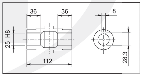
Eje hueco de salida / Hollow output shaft
